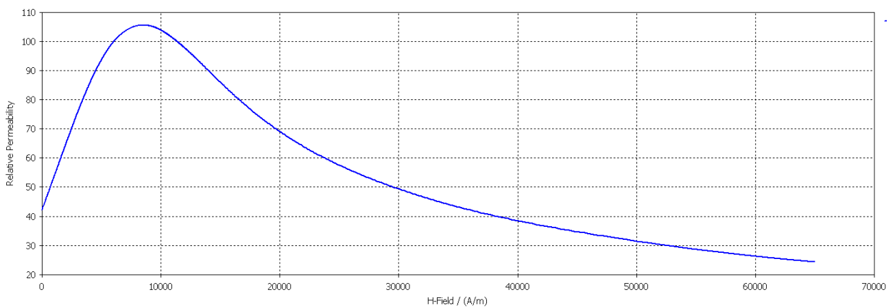
Figura 6: Permeabilità relativa non lineare del materiale costituente la fune metallica
