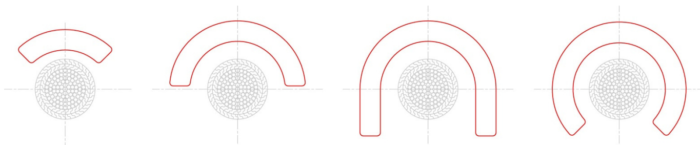
Figura 2: Disposizione dei sensori per detector di tipo "aperto"
