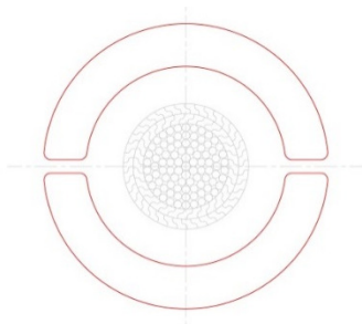
Figura 1 : Disposizione dei sensori per detector di tipo "chiuso "
