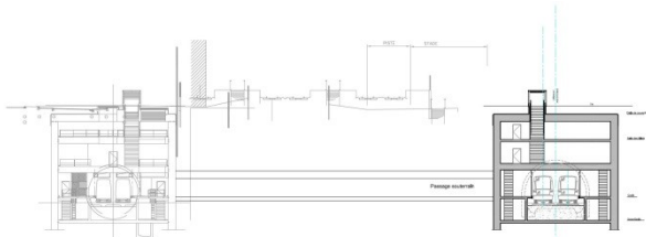
Profil en travers Projet Métro/ Subway Cross Section Project
