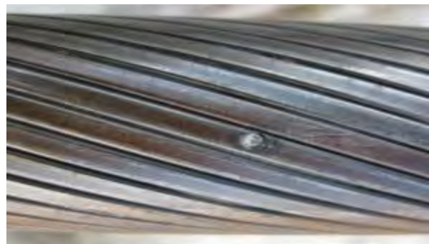
Abbildung 2.13: Kleiner Blitzschaden an VVS
