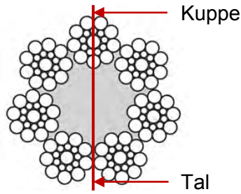
Abbildung 5.14: Seilquerschnitt bei ungerader Litzenzahl
