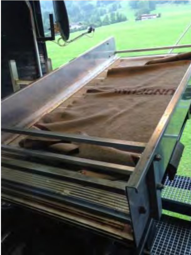
Abbildung 5.27: Liege zur visuellen Inspektion des Tragseiles an der Grüntenseilbahn
