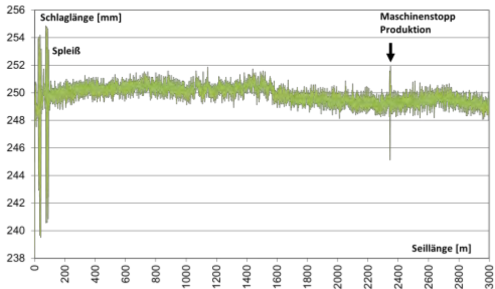
Abbildung 8.2: Sichtbarer Maschinenstopp aus der Produktion des Seils an einer kuppelbaren Einseilumlaufbahn
