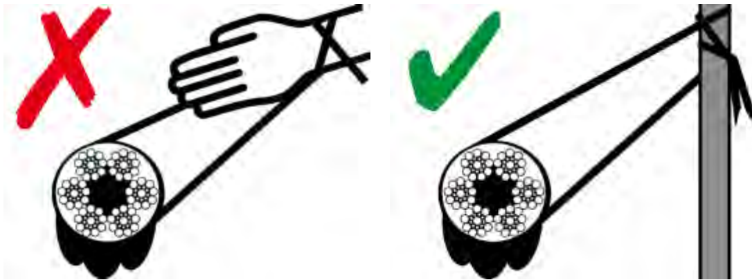
Abbildung 5.21: Empfohlene Befestigung eines Nylonstrumpfes
