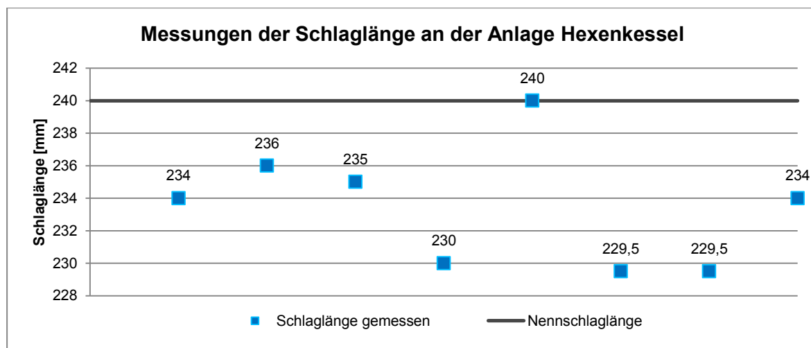
Abbildung 5.17: Messungen der Schlaglänge
