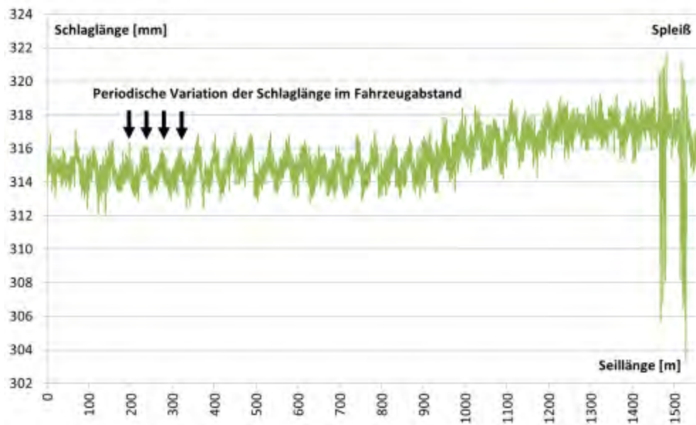
Abbildung 8.1: Drall an einer kuppelbaren Einseilumlaufbahn mit unzureichend gespurter Station – die Schlaglänge weist eine periodische Variation im Abstand der Fahrzeuge auf
