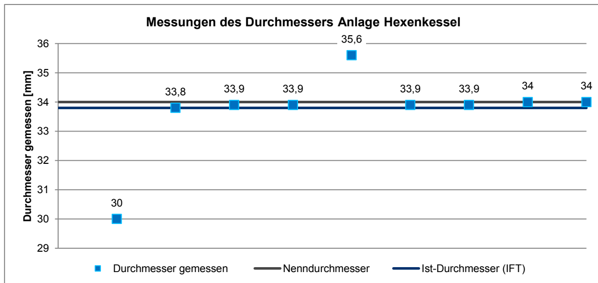
Abbildung 5.15: Messungen des Durchmessers an der Anlage Hexenkessel
