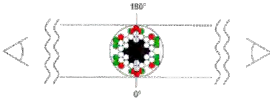
Abbildung 3.6: Sichtbarer Teil der Seiloberfläche bei der visuellen Seilinspektion
