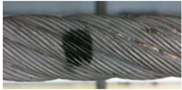
Abbildung 4.16: Drahtbruch 1,5 x Litzen- durchmesser
