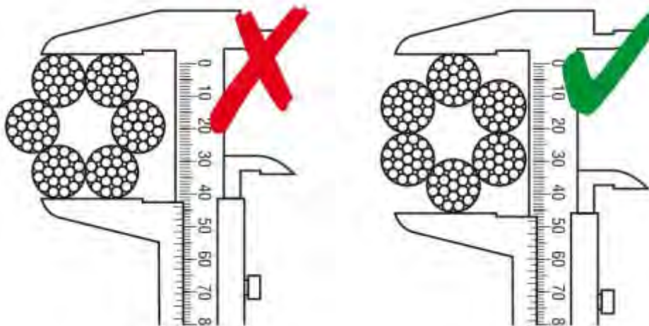
Abbildung 5.13: Korrekte Messung des Seildurchmessers [9]
