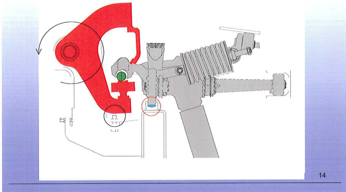
Bild 14: Zwangskuppelapparat ausgelenkt
